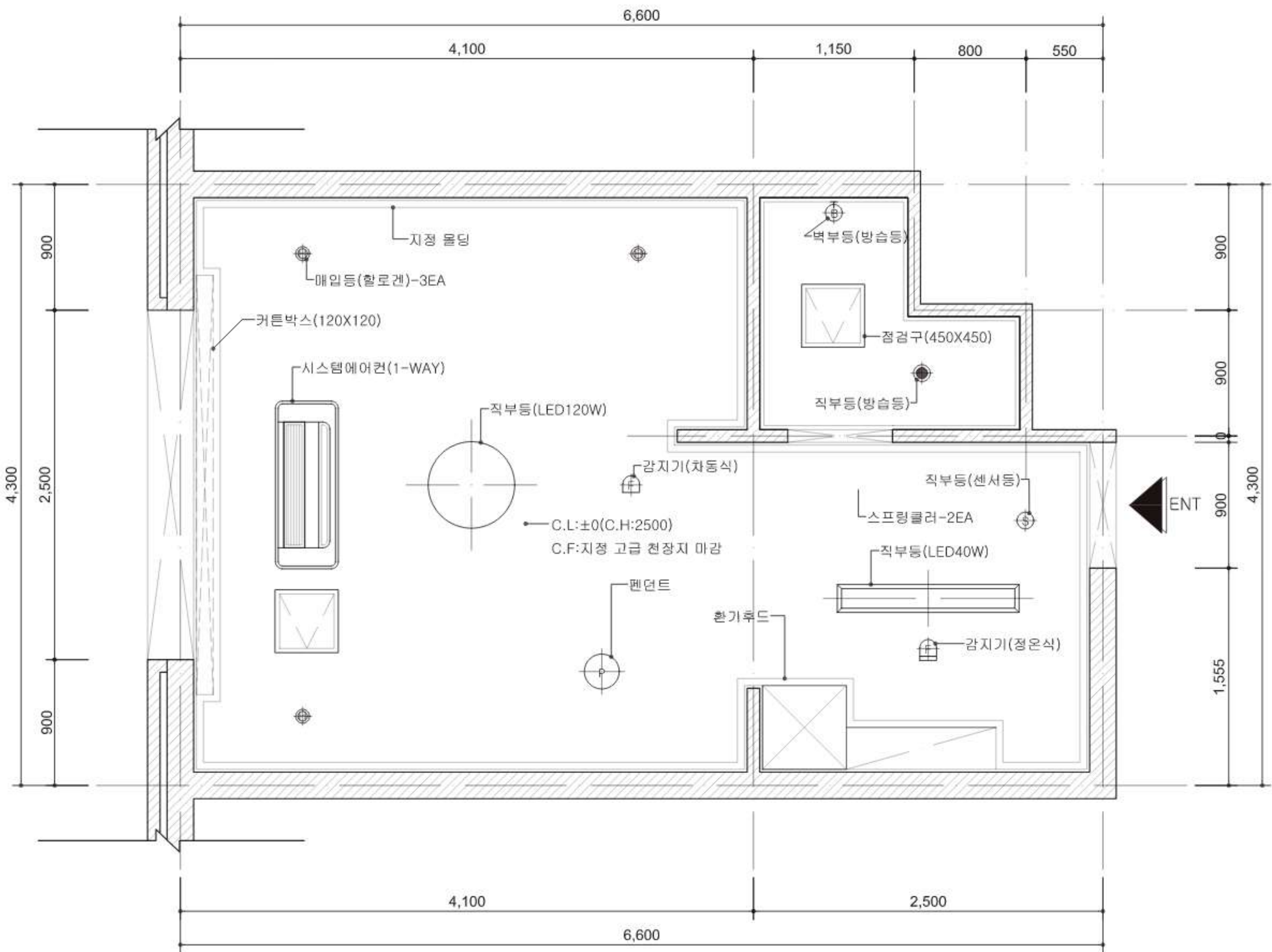
원룸 천장도 SCALE: 1/50
