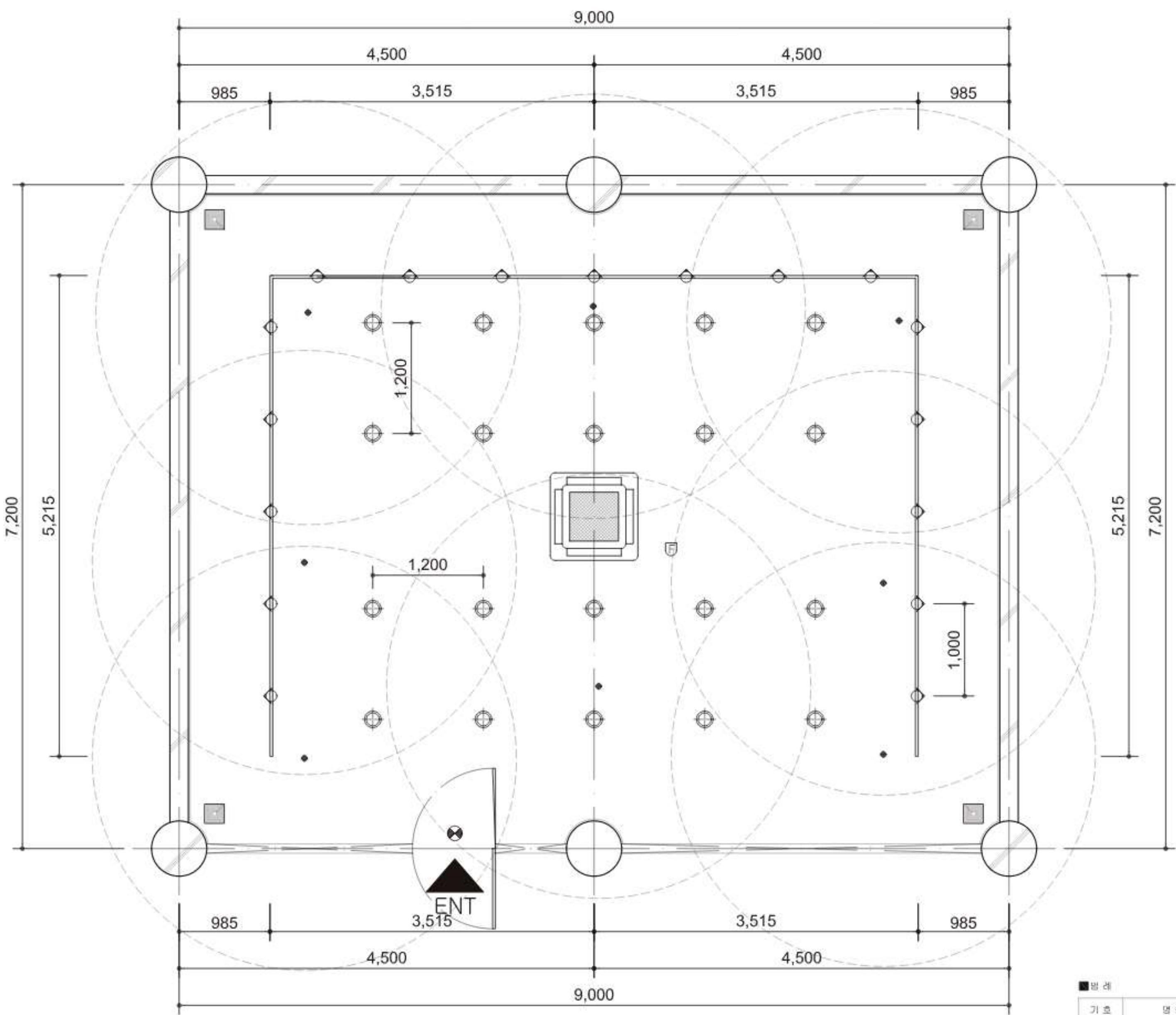
천장도 SCALE:1/50
