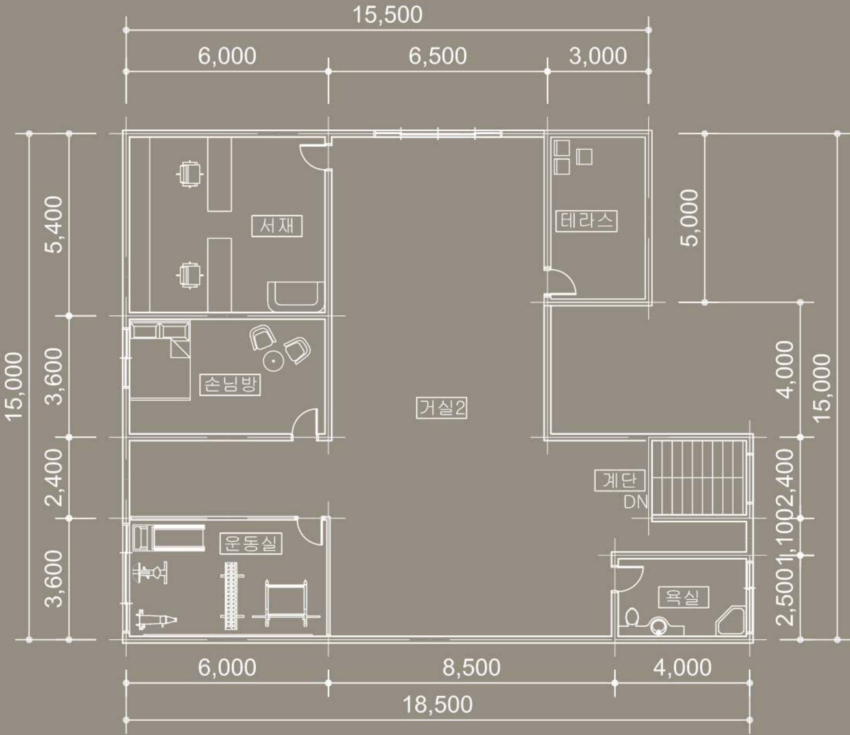
2층 평면도 SCALE: 1/120
