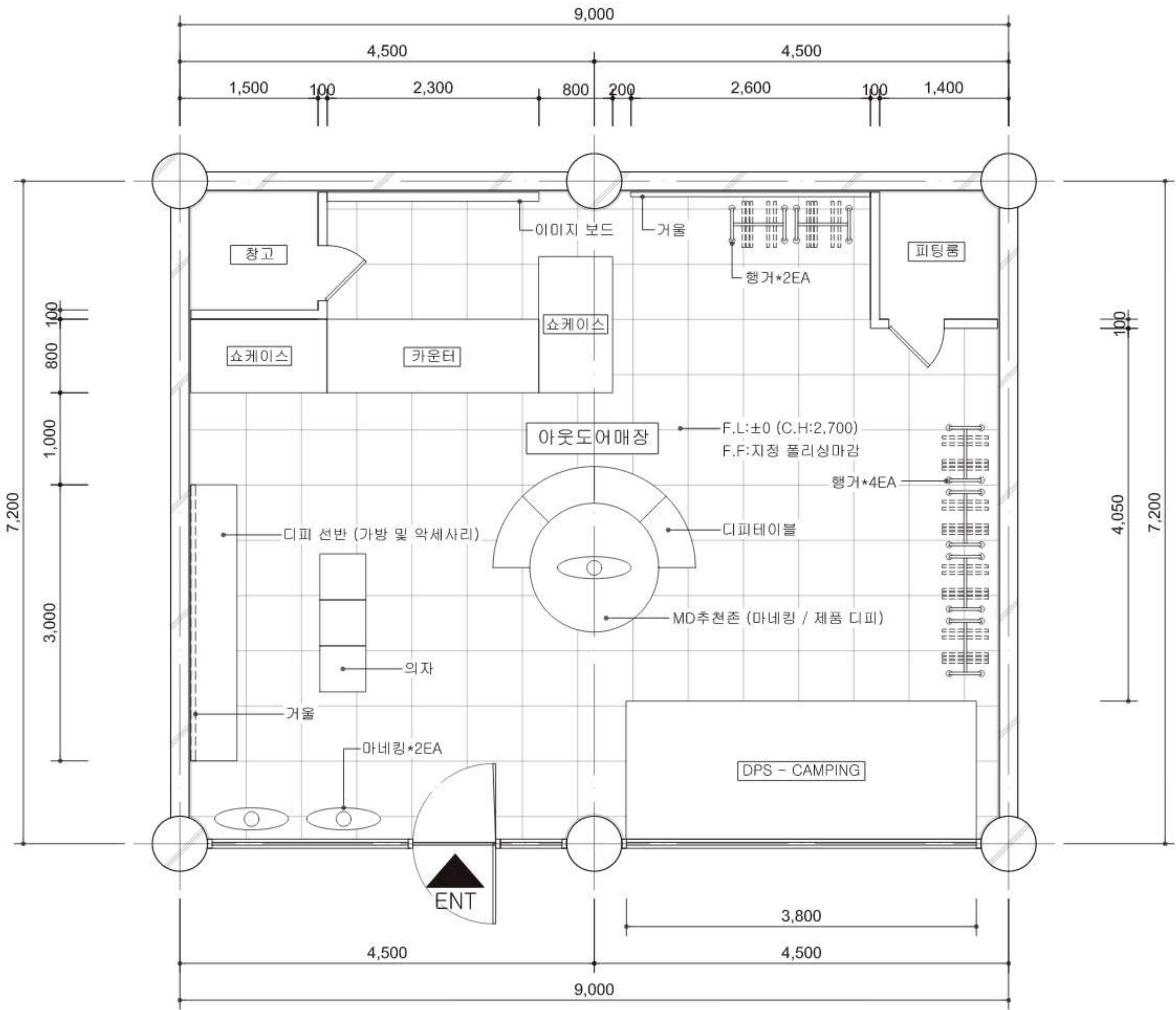
평면도 SCALE:1/50
