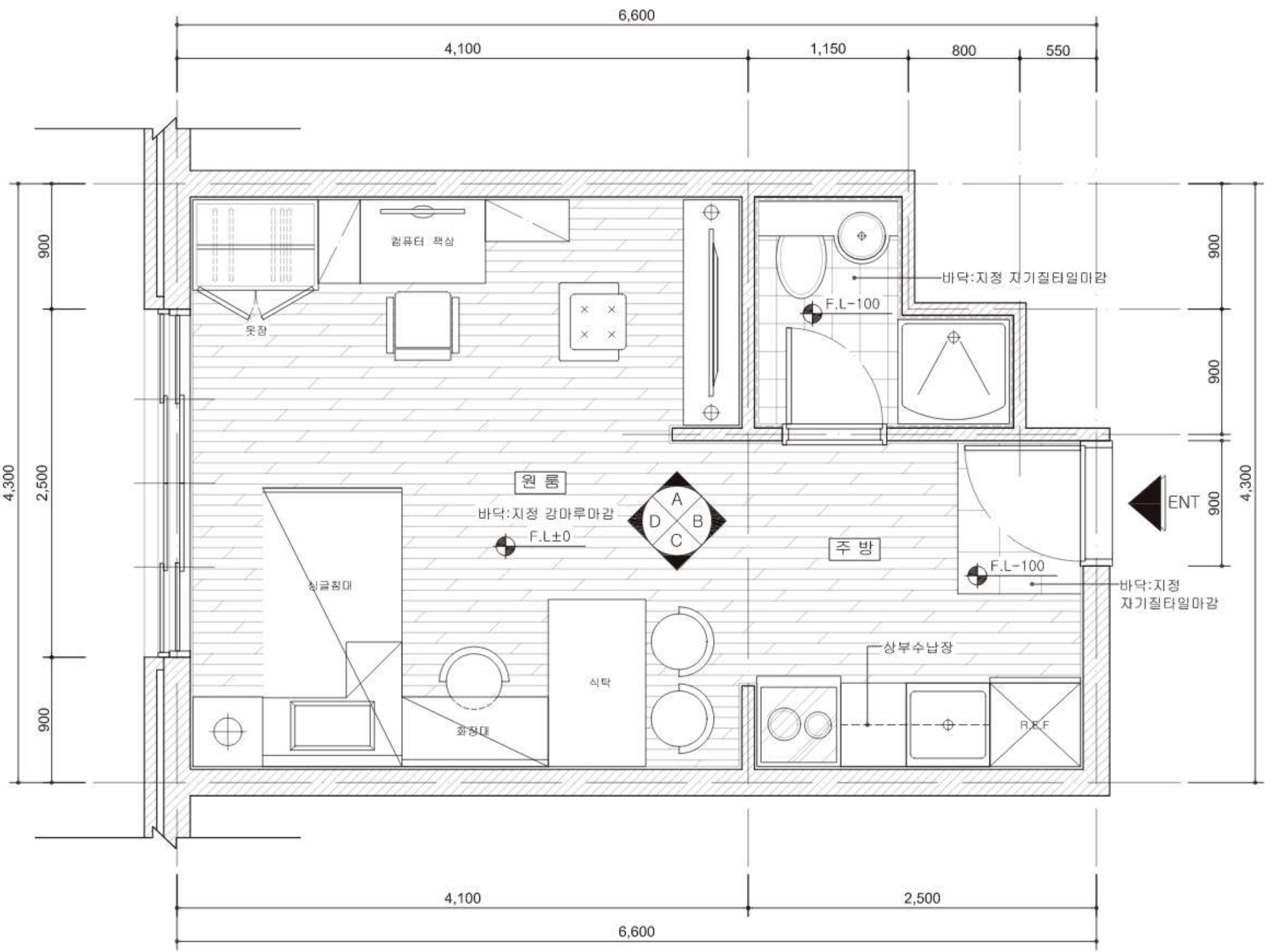
원룸 평면도 SCALE: 1/30
