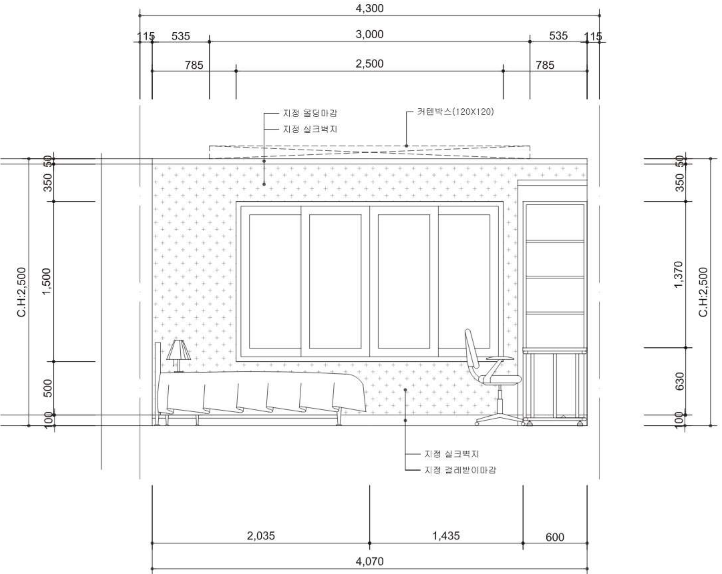
실 내 입 면 도 -D SCALE: 1/50
